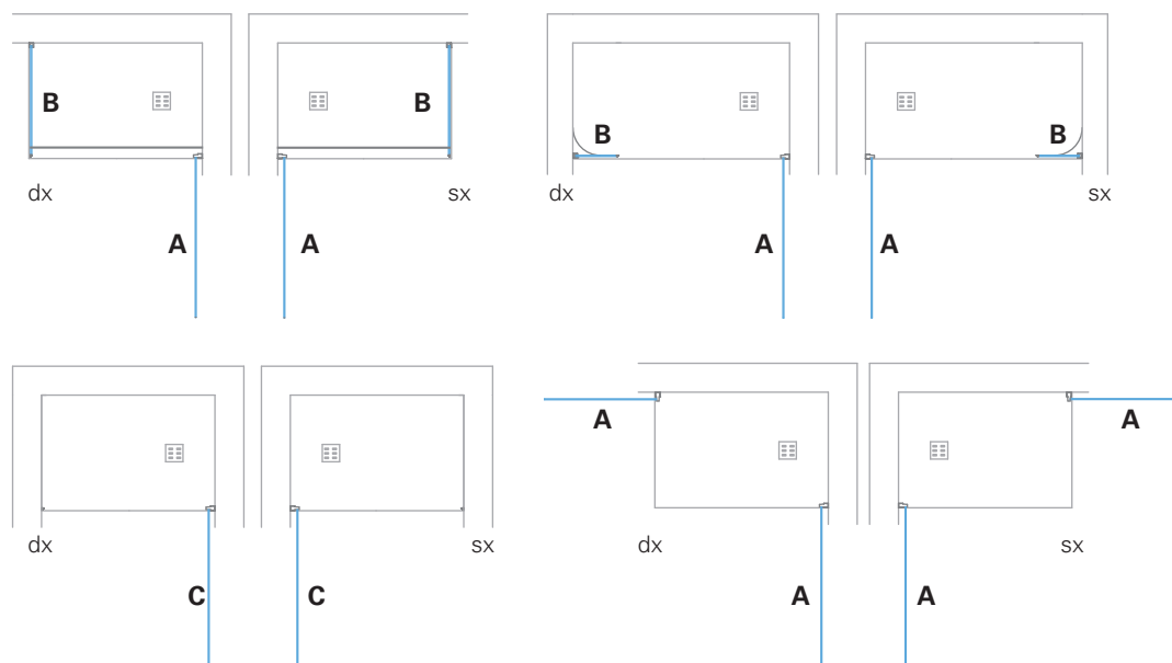
Cerniera superiore / Upper hinge
